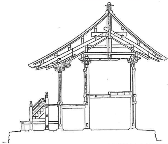
富士浅間宮本殿断面図
